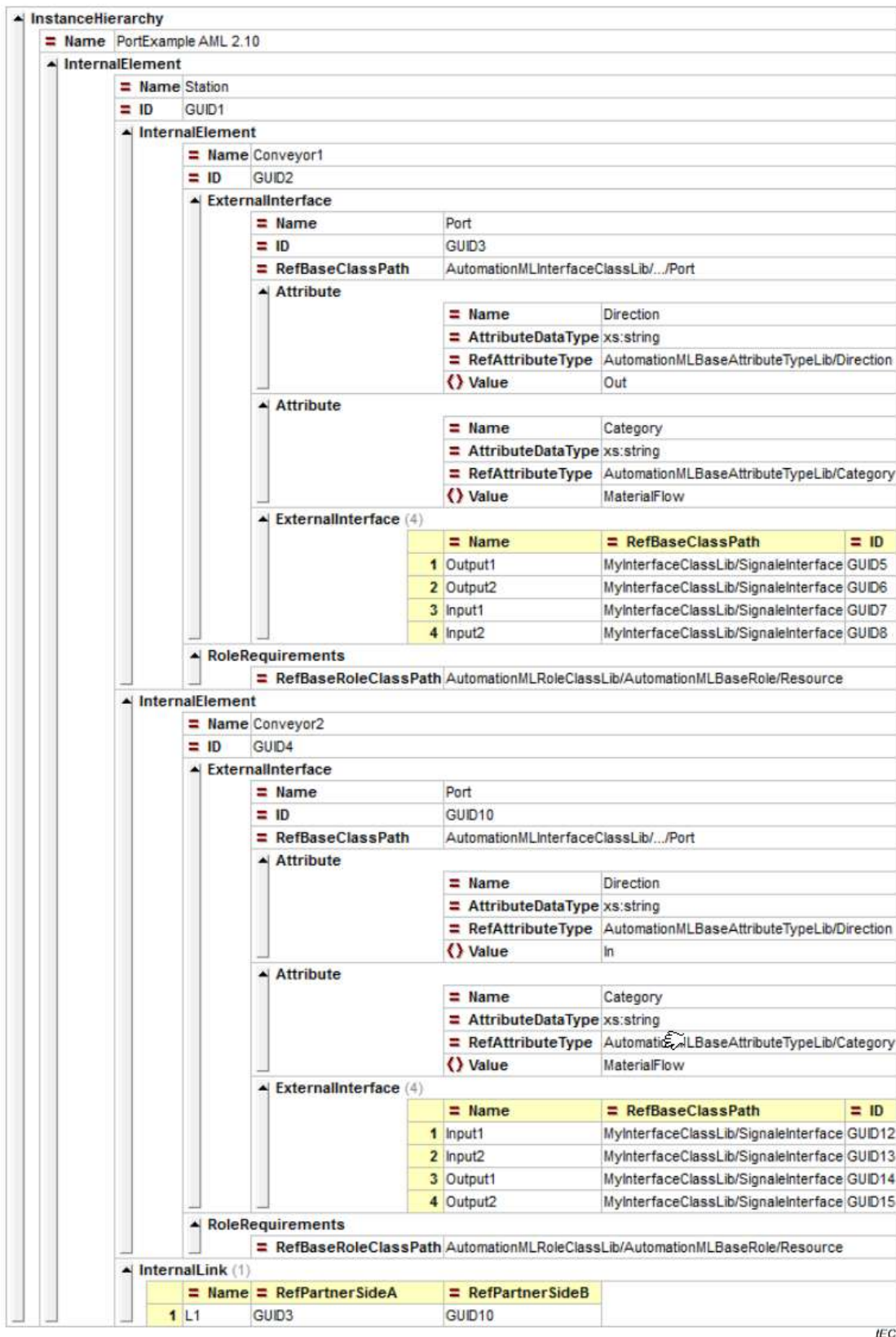
图A.15 AML 端口概念的 XML 描述
