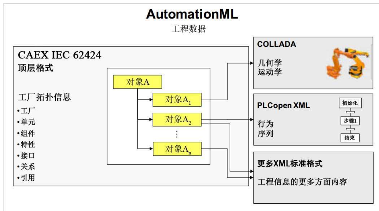
图A.1 AML通用架构
