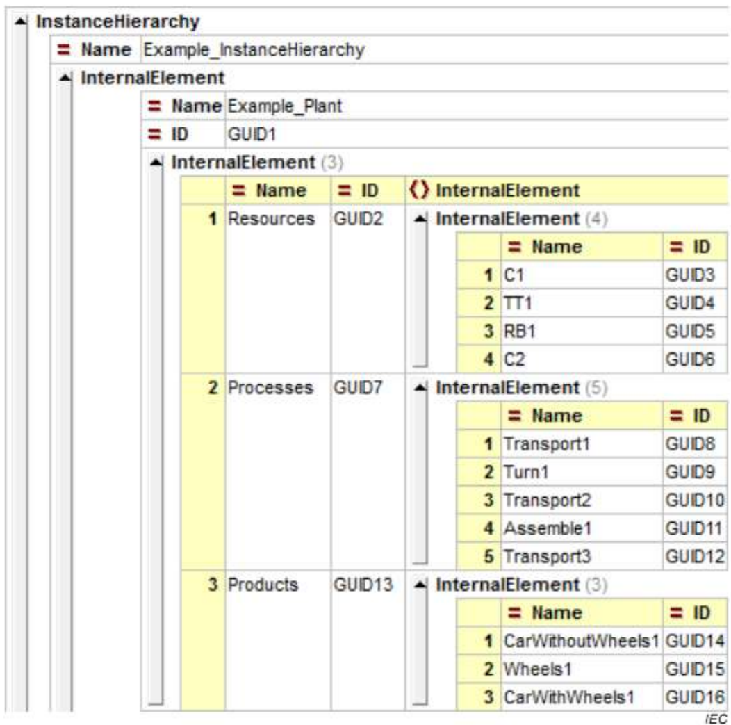
图A.34 示例中的内部元素
