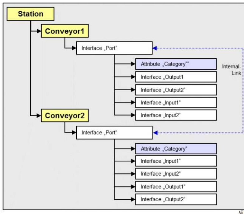
图A.14 描述 AML 端口概念的示例
