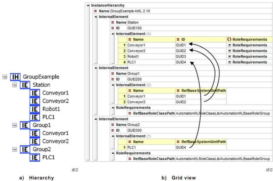
图A.20 AML 组示例-对象树、表格视图
