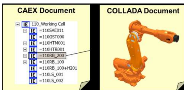
图A.3 CAEX 文档对 COLLADA 文档的引用
