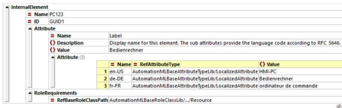
图A.38 AML 多语言表达概念 XML 描述
