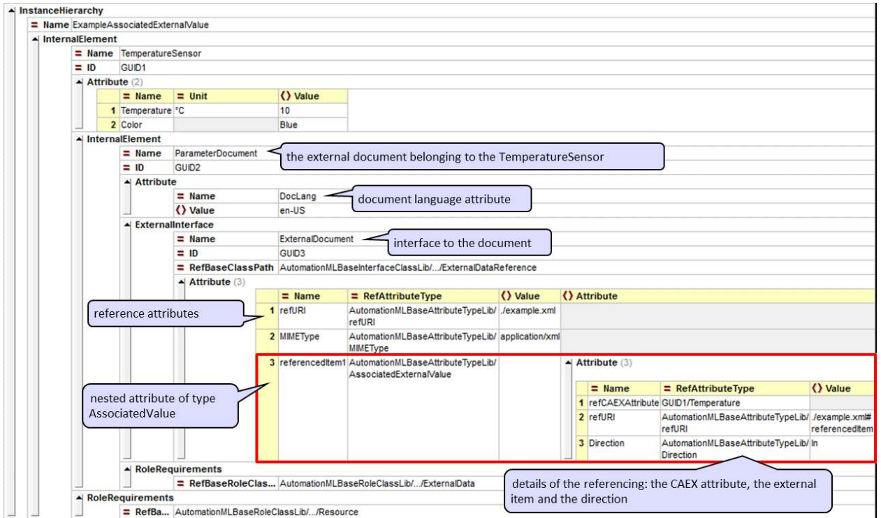
图A.7 CAEX 属性引用到外部文档项的示例
