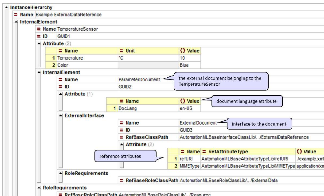
图A.5 引用外部文档示例
