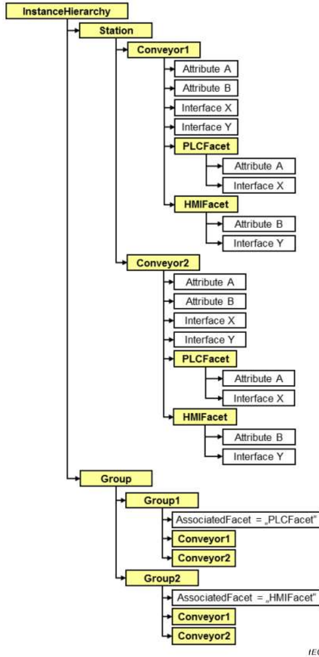
图A.22 面概念与组概念的组合
