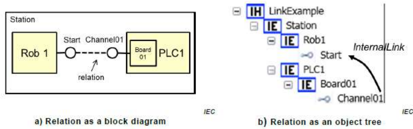
图4 关系表示例-框图、对象树
