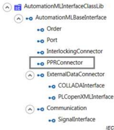
图A. 27 PPR 连接器接口
