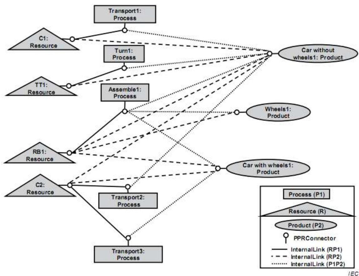
图A.31 示例中的链接
