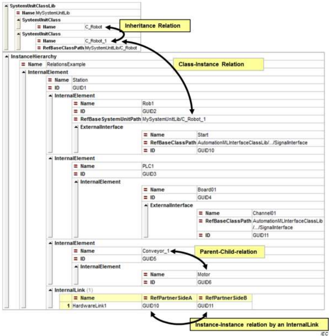
图A.10 关系示例的 XML 描述
