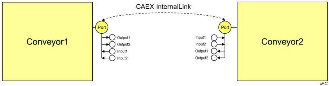
图A.13 端口概念
